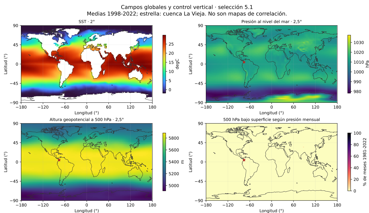
Figura 34: Campos obtenidos y control vertical; no son mapas de correlación.
